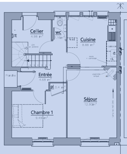
Rez-de-chaussée :
